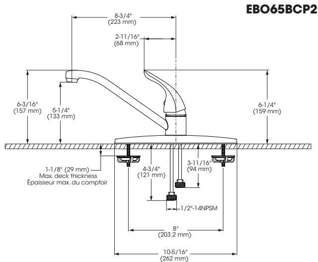
EBO65BCP2
